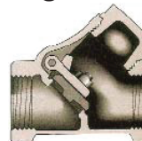
Fig. 36 Y Swing Check
