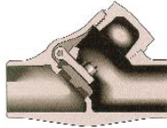
Fig. 1342S Y Check
